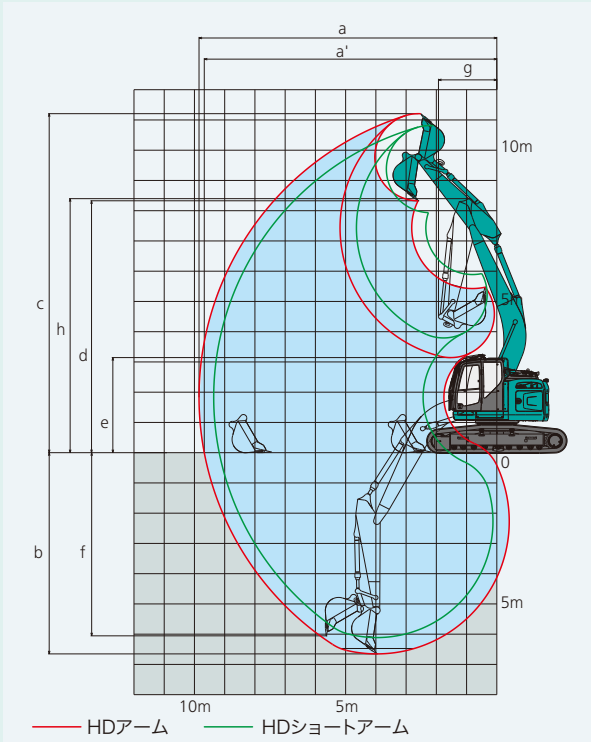
■作業範囲図 (図はSK235SRD-5)
