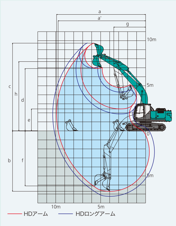
■作業範囲図 (図はSK210D-10)
