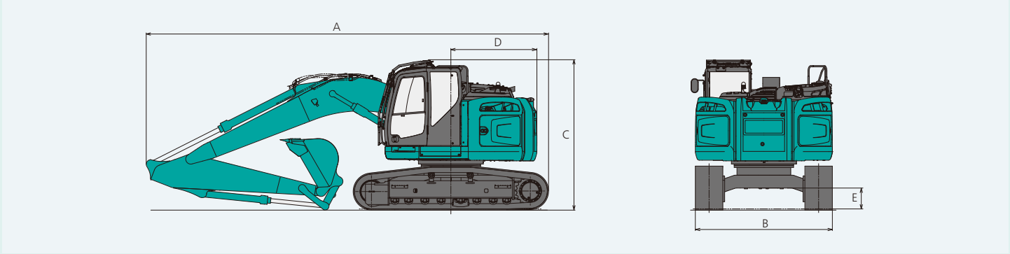
■全体図 (図はSK235SRD-5)
