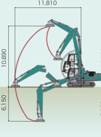
ストレートブーム(7.50m)仕様
