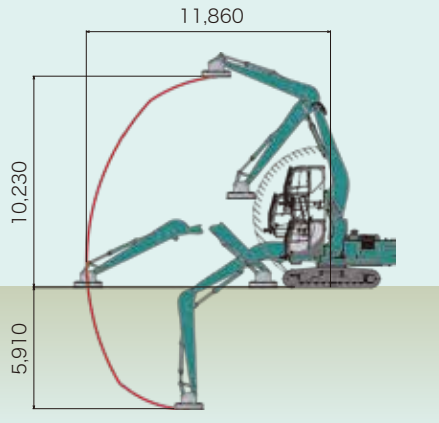
ベンドブーム(6.90m)・5.05mアーム仕様
