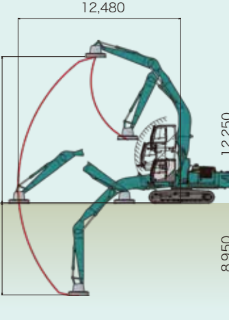
ベンドブーム(8.20m)仕様
