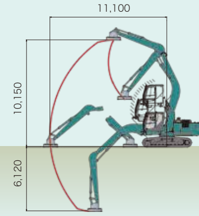
スクラップローダ・4.90mアーム仕様
