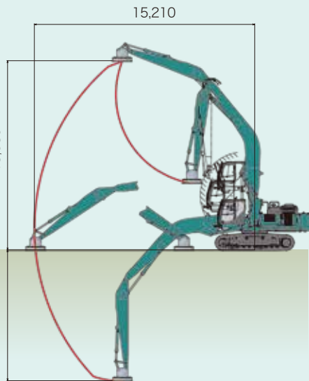
ベンドブーム(9.70m)仕様
