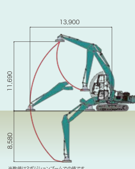
ベンドブーム(8.30m)仕様
