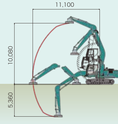
ベンドブーム(6.90m)・QH配管付き専用ショートアーム(4.50m)仕様
