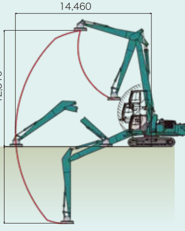
ストレートブーム(9.30m)仕様
