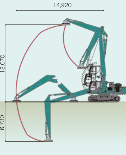
ストレートブーム(9.30m)仕様
