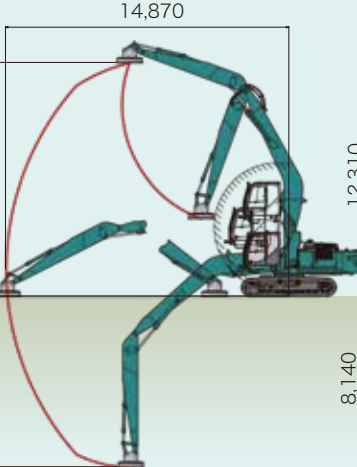
ベンドブーム(8.90m)仕様
