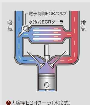
③ 大容量EGRクーラ(水冷式)
