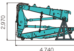
■3つ折れ超ロングアタッチメント
