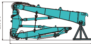
■3つ折れ超ロングアタッチメント
