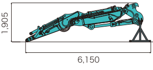
■セバレートブームアタッチメント
