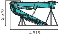
■2つ折れ超ロングアタッチメント
